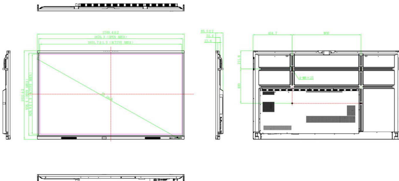
75": ST-75-CONNECT-PRO5
