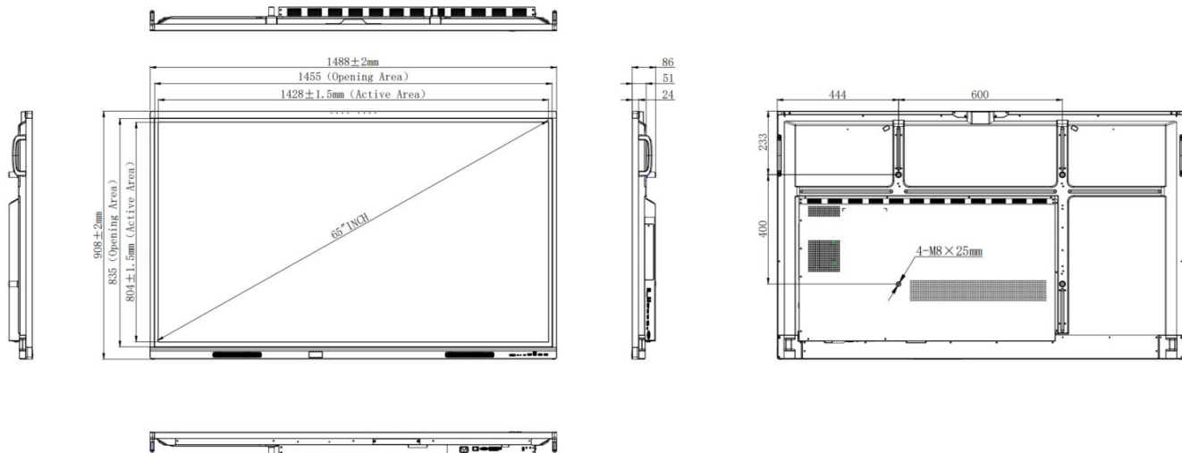
65": ST-65-CONNECT-PRO5
