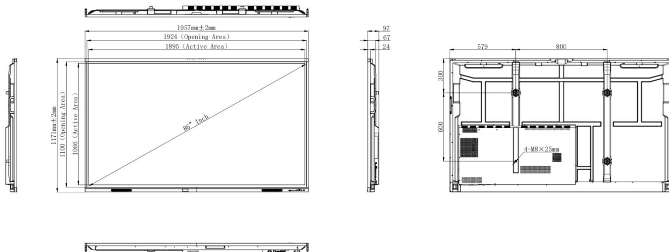
86": ST-86-CONNECT-PRO5
